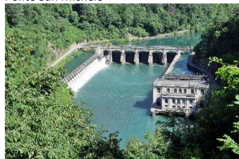
Centrale Semenza, Diga e Presa del Canale Edison
